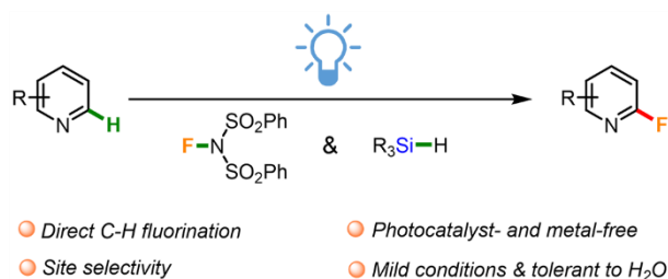
图 1 可见光诱导氮杂芳烃碳氢键选择性氟化反应
